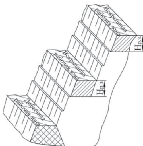
Рис. 1. Схема распределения рабочих зон при отработке крутонаклонными слоями: H_{p.з.} – высота обрабатываемой рабочей зоны (может соответствовать высоте уступа)
