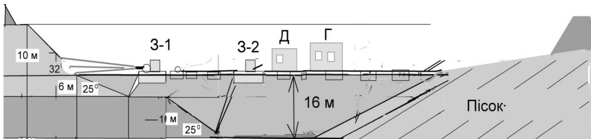
Рис. 2. Профіль кар'єру з плавучою фабрикою. 3-1, 3-2 – розкривний і видобувний земснаряди, Д – установка дешламації, Г – установка гравітаційного збагачення
