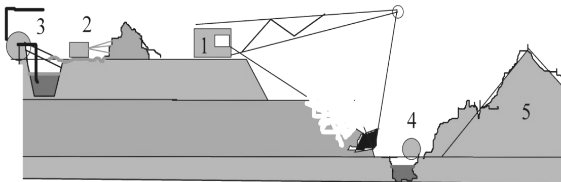
Рис.1. Технологія відробки родовищ Іршанської групи. 1 – драглайн, 2 –монітор, 3 – ґрунтовий насос, 4 – насос водовідливу, 5 – внутрішній відвал
