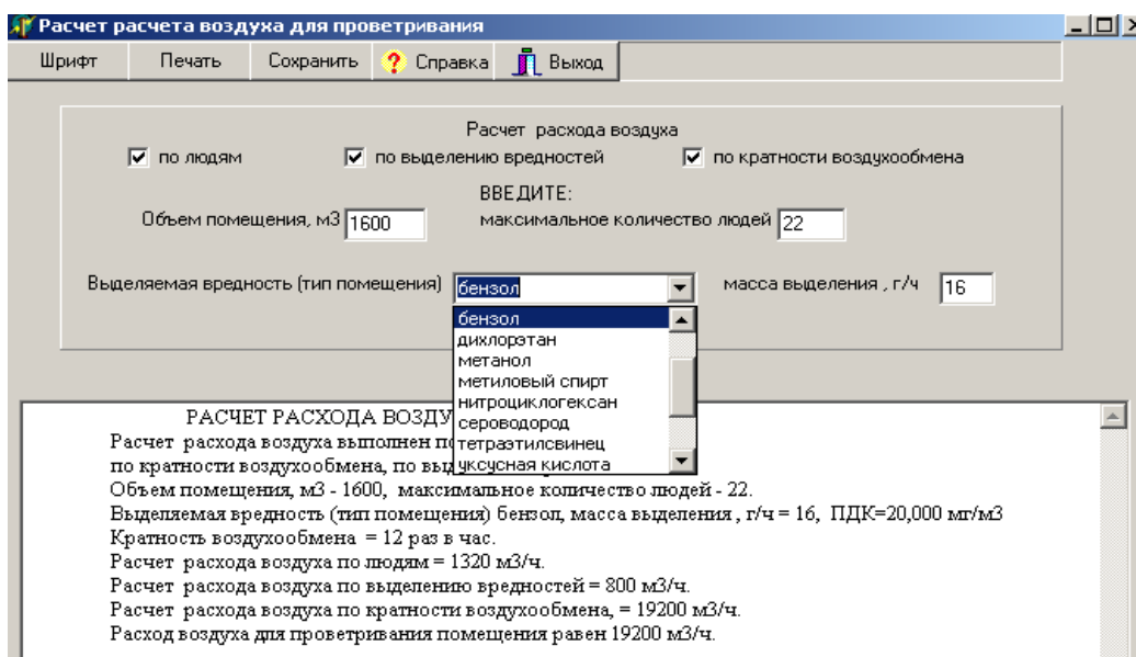
Рис. 1. Вікно розрахунку витрат повітря
