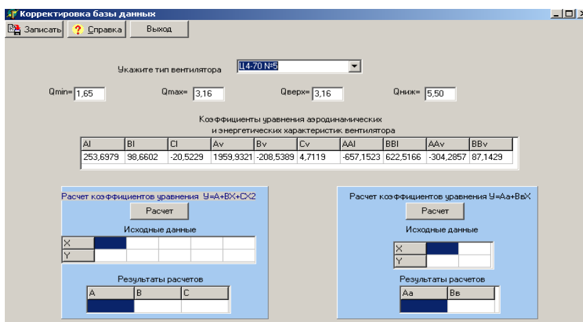
Рис. 5. Вікно корегування БД
