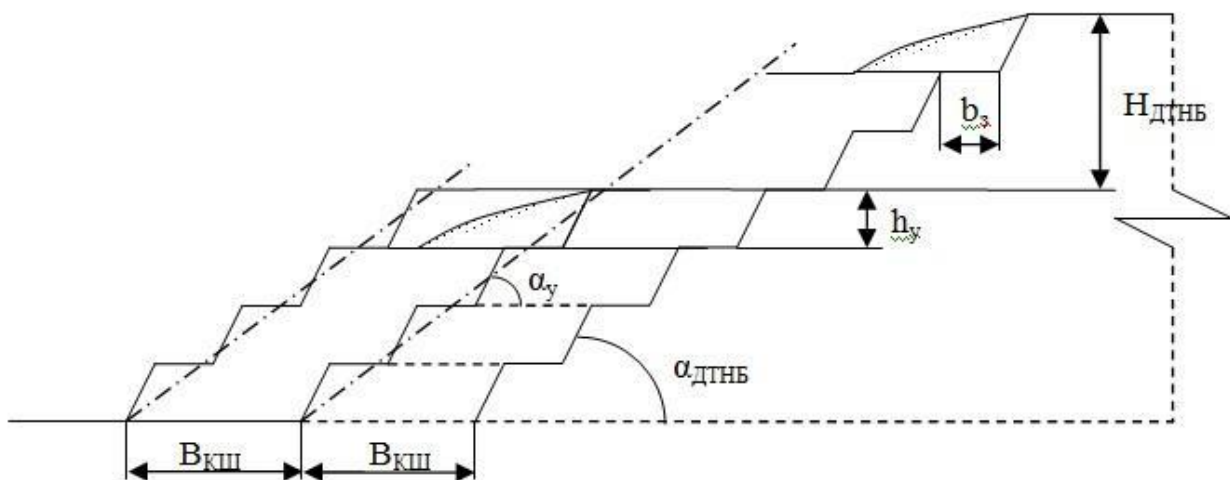
Рис.2. Схема відпрацювання борту крутими виймальними шарами
